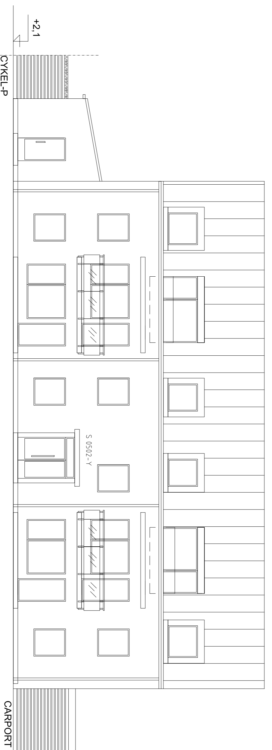
FASAD MOT NORDVÄST, GÅRD
